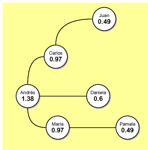
Figura 4: Centralidad c(0,5) .
